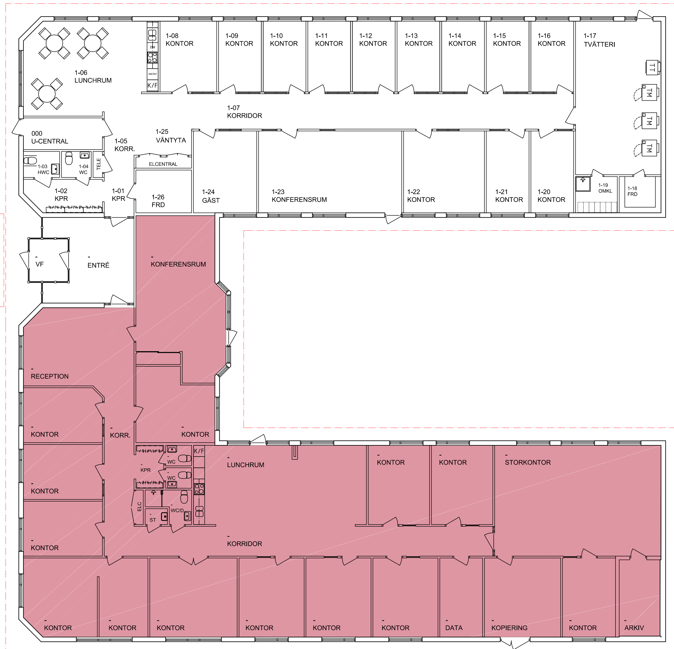
PLAN, BOTTENVÅNING
